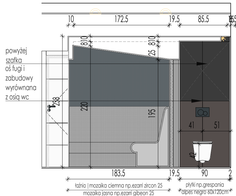
WIDOK H-H
