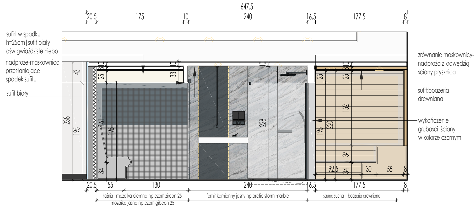
WIDOK E-E
