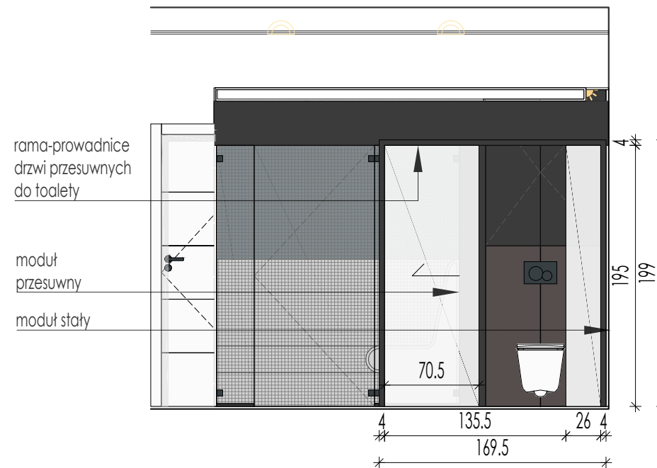
WIDOK G-G Z DRZWIAMI PRZESUWNymi DO TOALETY
