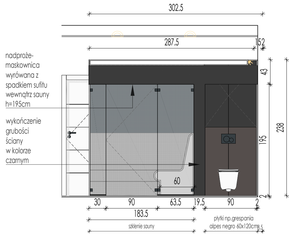
WIDOK G-G
