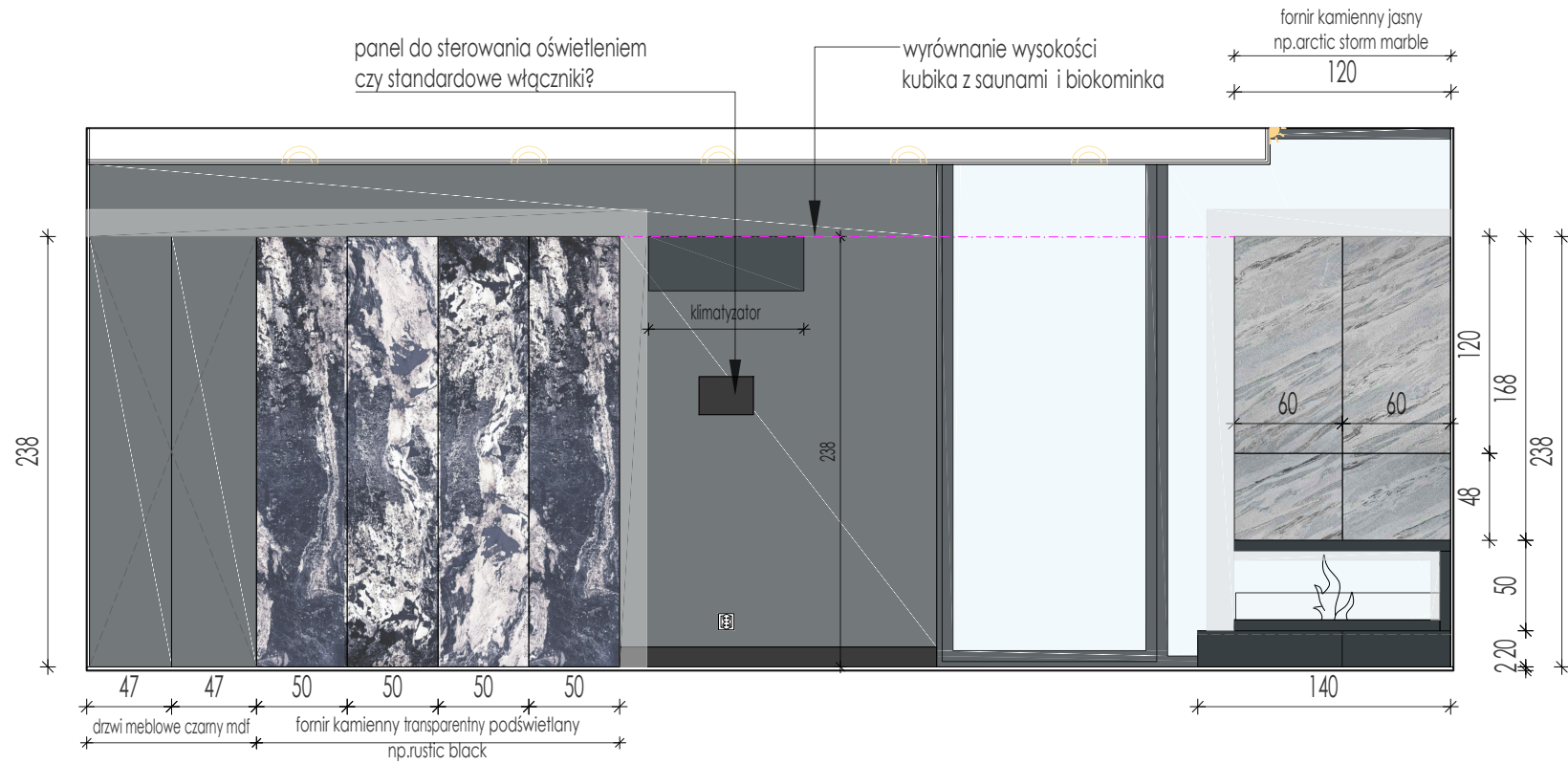
WIDOK B-B
